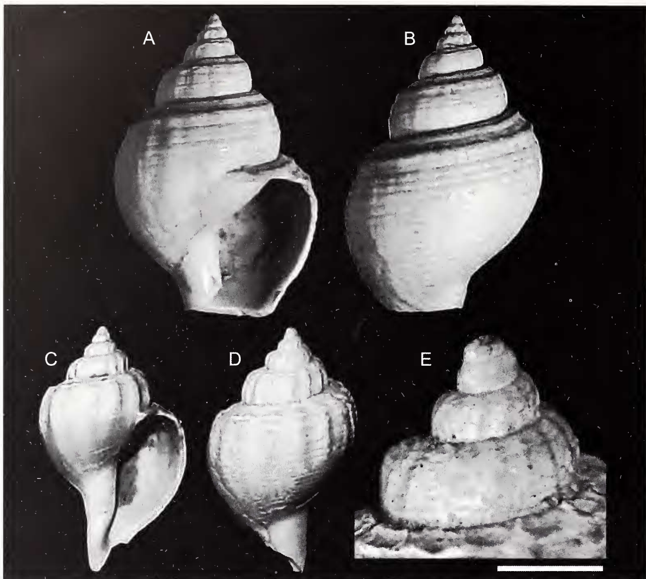
Fig. 13. Admete viridula (Fabricius, 1780) A, B. Codrignano (Imola, Bologna), Santerniano, H = 15,5 mm (coll. Della Bella) C, D. Codrignano (Imola, Bologna), Santerniano, H = 9,4 mm (coll. Della Bella). E. Particolare dei primi giri Codrignano (Imola, Bologna), Santerniano (coll. Della Bella). Scala = 1 mm.
